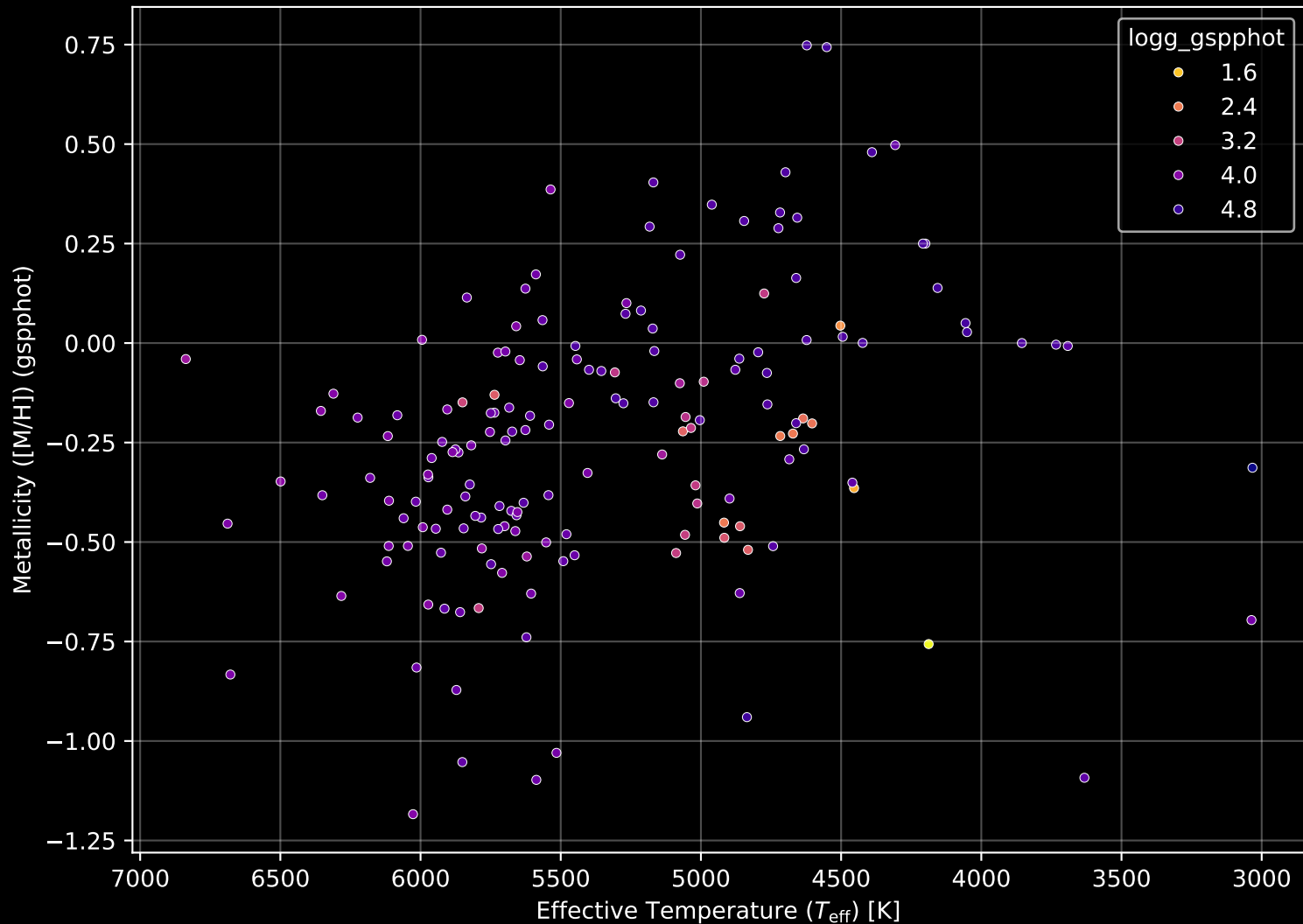
APOGEE DR17 Field: [103+81_MGA] Stellar Population Parameters (n= 166)
